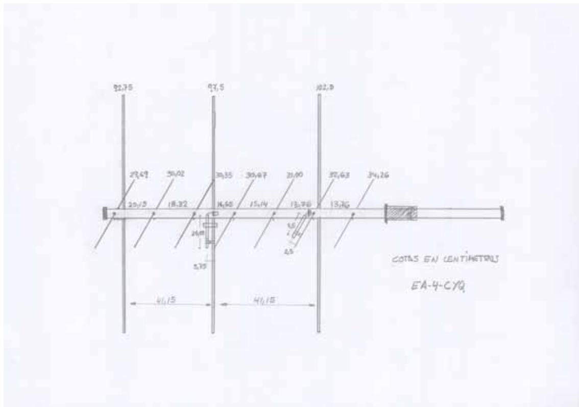
Figura n°1: Esquema de antena bibanda portable
